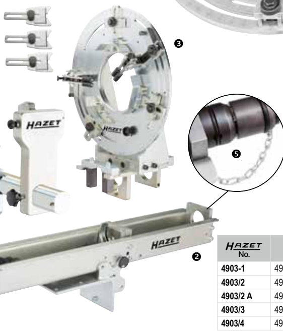
Mocowanie kolumny McPhersona
